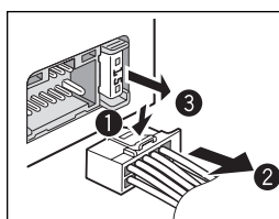
Соединитель антенны радиоприемника (RADIO ANT IN)
